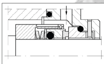
NV-3.1 Углеродистый, запрессованный во вращающееся кольцо
