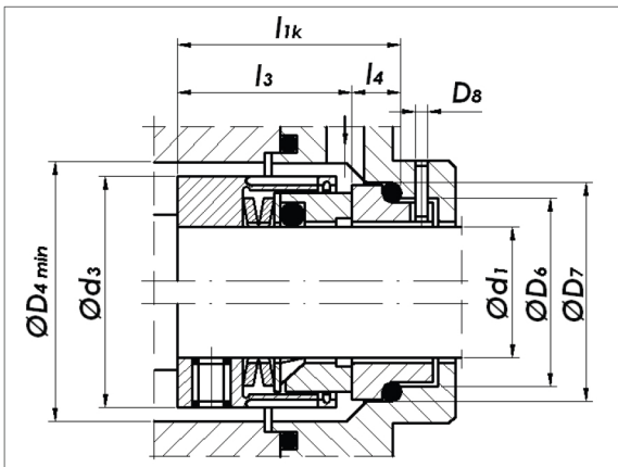
NV-3.1 Углеродистый, запрессованный во вращающееся кольцо
